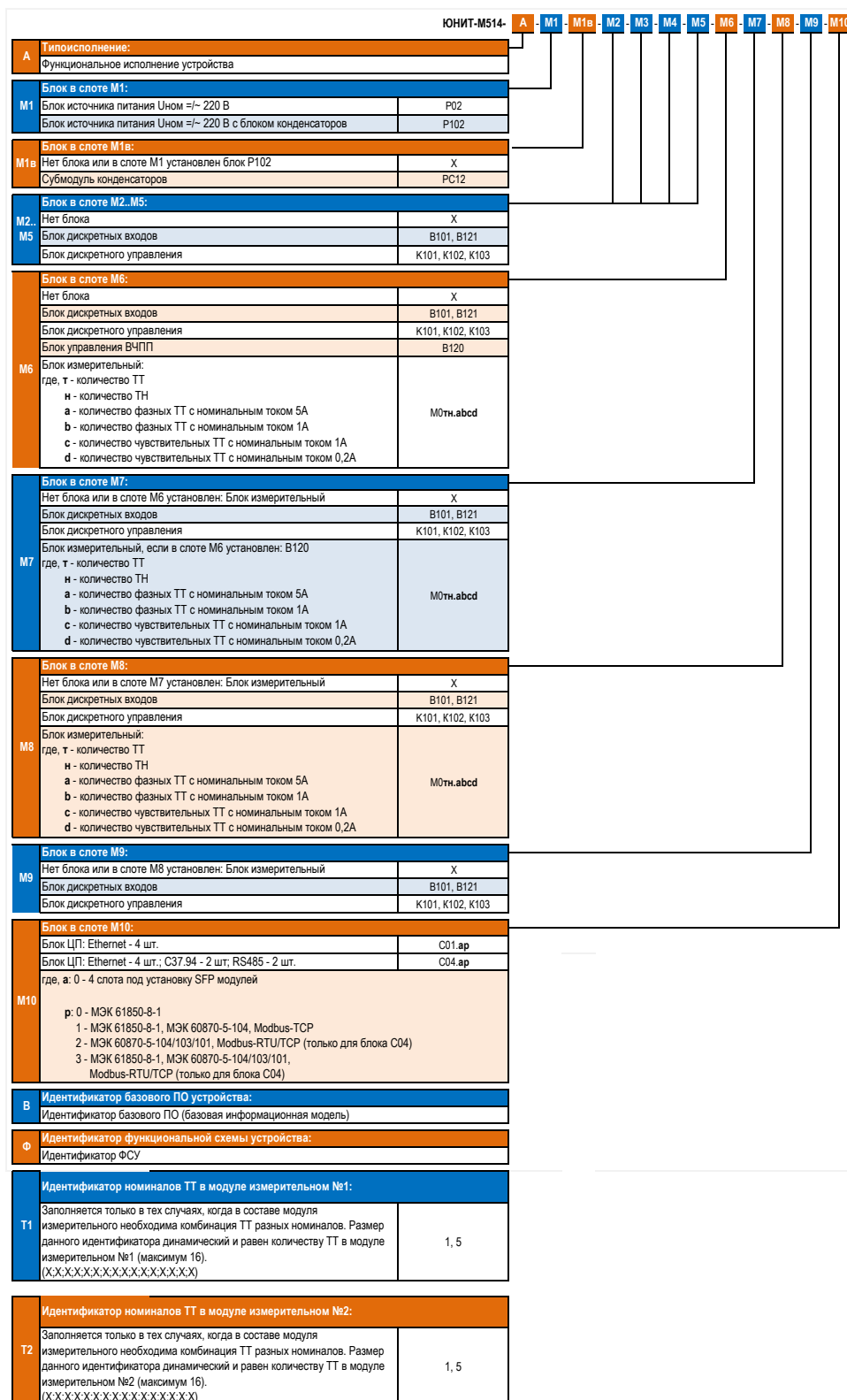
Приложение А (обязательное) Код заказа устройства «ЮНИТ-М514»
